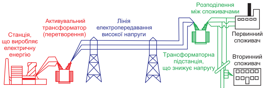
Мал. 25.3. Схема виробництва електроенергії та забезпечення споживачів
