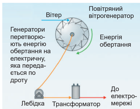
Мал. 54.2. Літальна ВЕС
