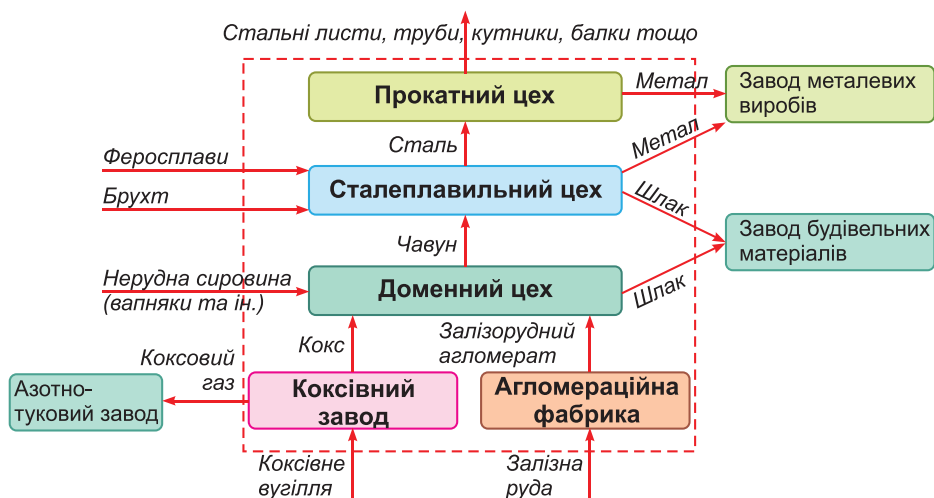
Мал. 27.2. Схема металургійного комбінату повного циклу
